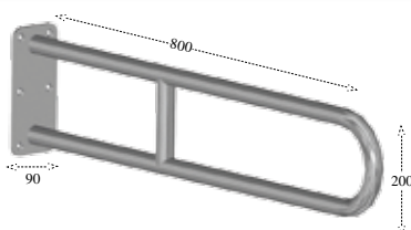
MN-015 (nerez) pevné madlo k WC 1 991,-
