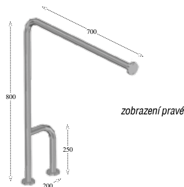
MN-018 (nerez) pevné madlo k WC (pravé i levé) 2 510,-
