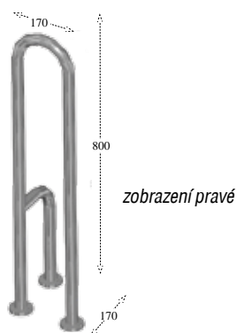
MN-009 (nerez) madlo k WC (pravé i levé) 2 510,-
