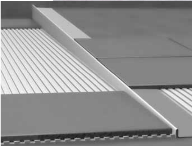
Zobrazeno provedení pravé (p)
