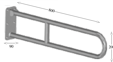
MN-008 (nerez) sklopné madlo 2 451,-
